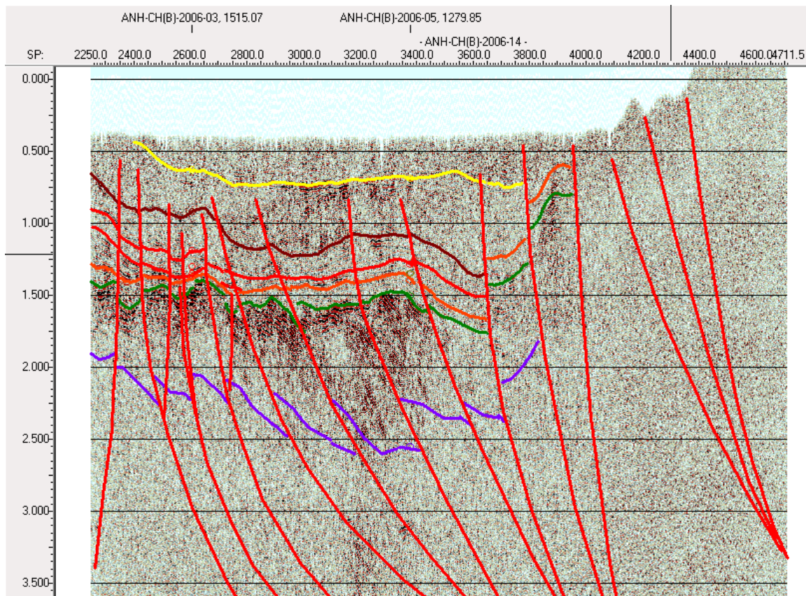
Figura 15. Sección sísmica ANH-CHOCO - 2006-14 migrada tiempo
