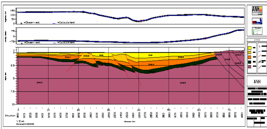
Figura 5. Perfil Gravimétrico de la línea ANH-CH(B)-2006-12
