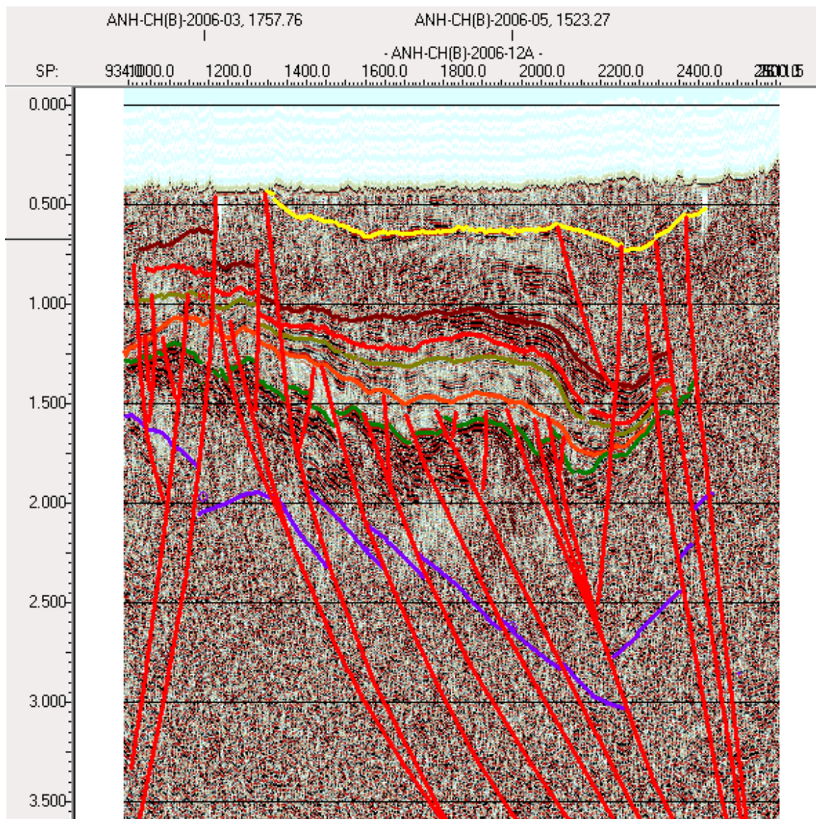
Figura 17. Sección sísmica ANH-CH(B)-2006-12A Migrada en tiempo.
