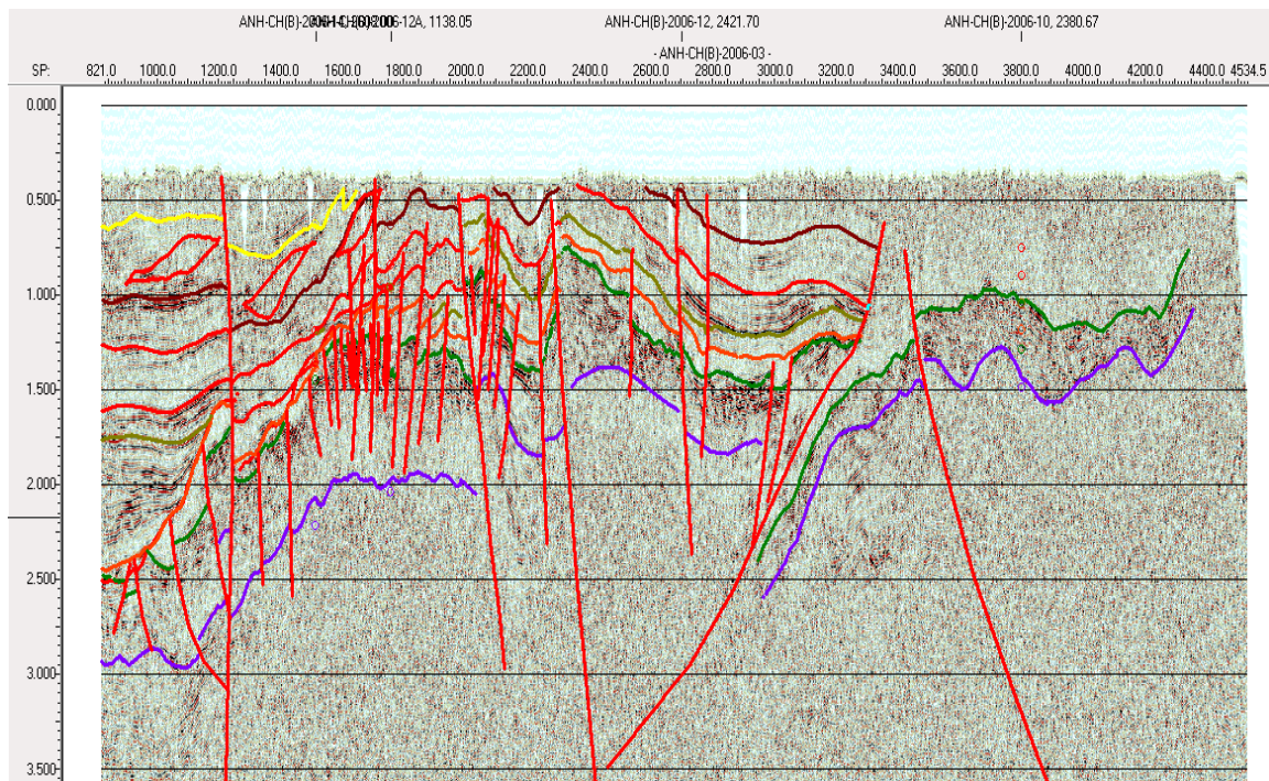
Figura 13. Sección sísmica ANH-CHOCO-2006-03 Migrada en tiempo
