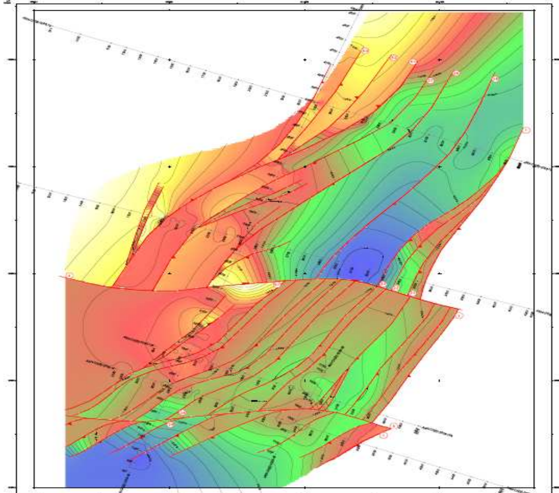
Mapa 20. Mapa estructural tope Cretáceo-Paleoceno TWT IC: 100 Mlsg. Datum: 500 metros SNM.
