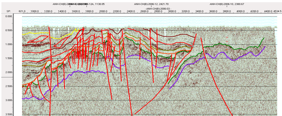
Figura 10. Sección sísmica ANH-CHOCO-2006-03
