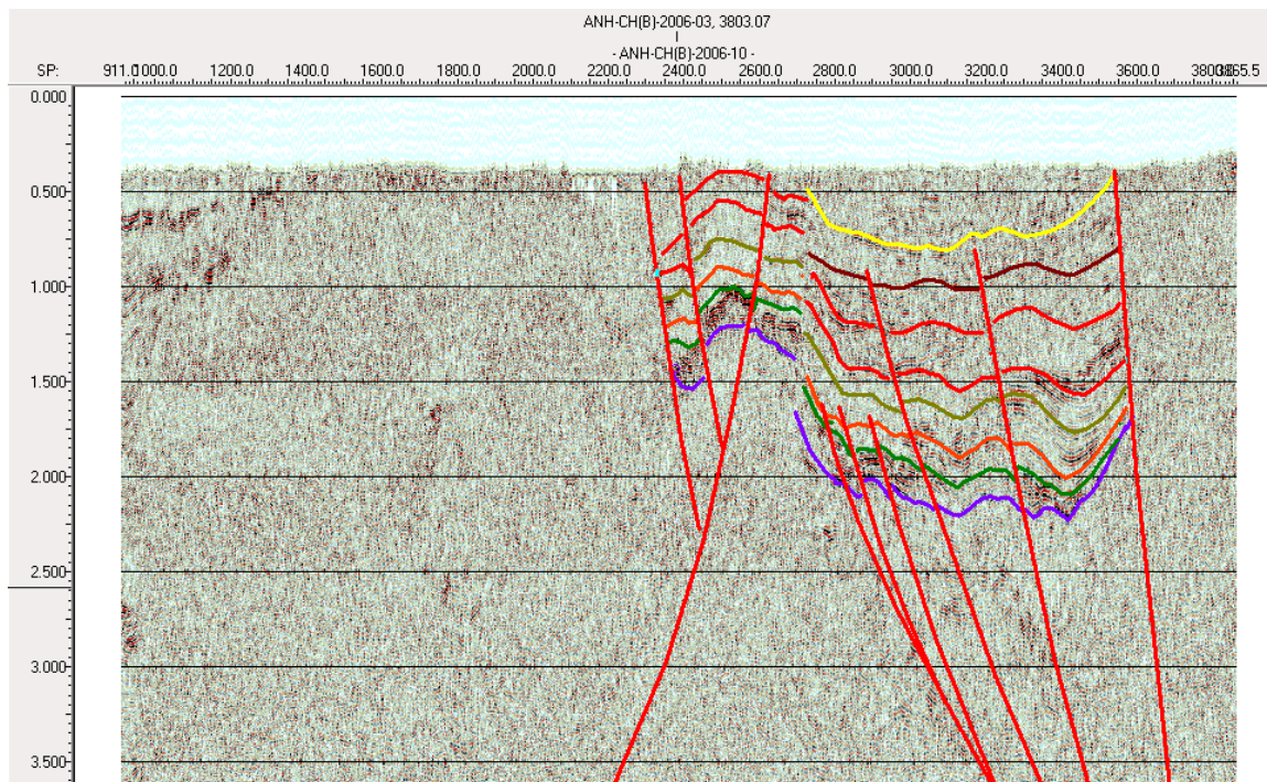
Figura 16. Sección sísmica ANH-CHOCO-2006-10 migrada en tiempo
