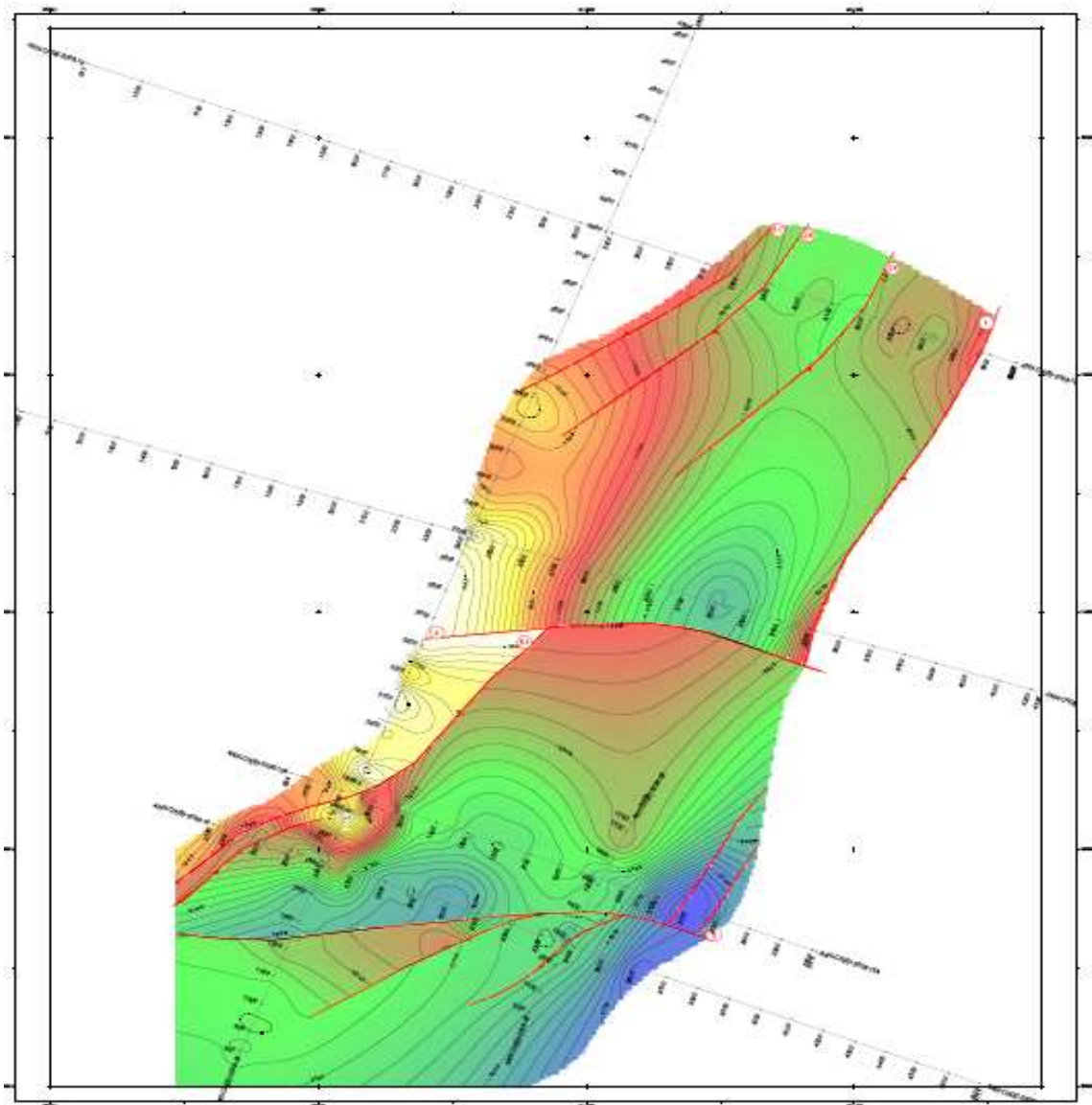
Figura 29. Mapa estructural tope del Grupo San Juan IC: 200 pies
