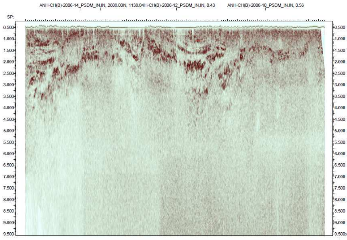
Sección ANH-CH(B)-2006-03 PSDM
