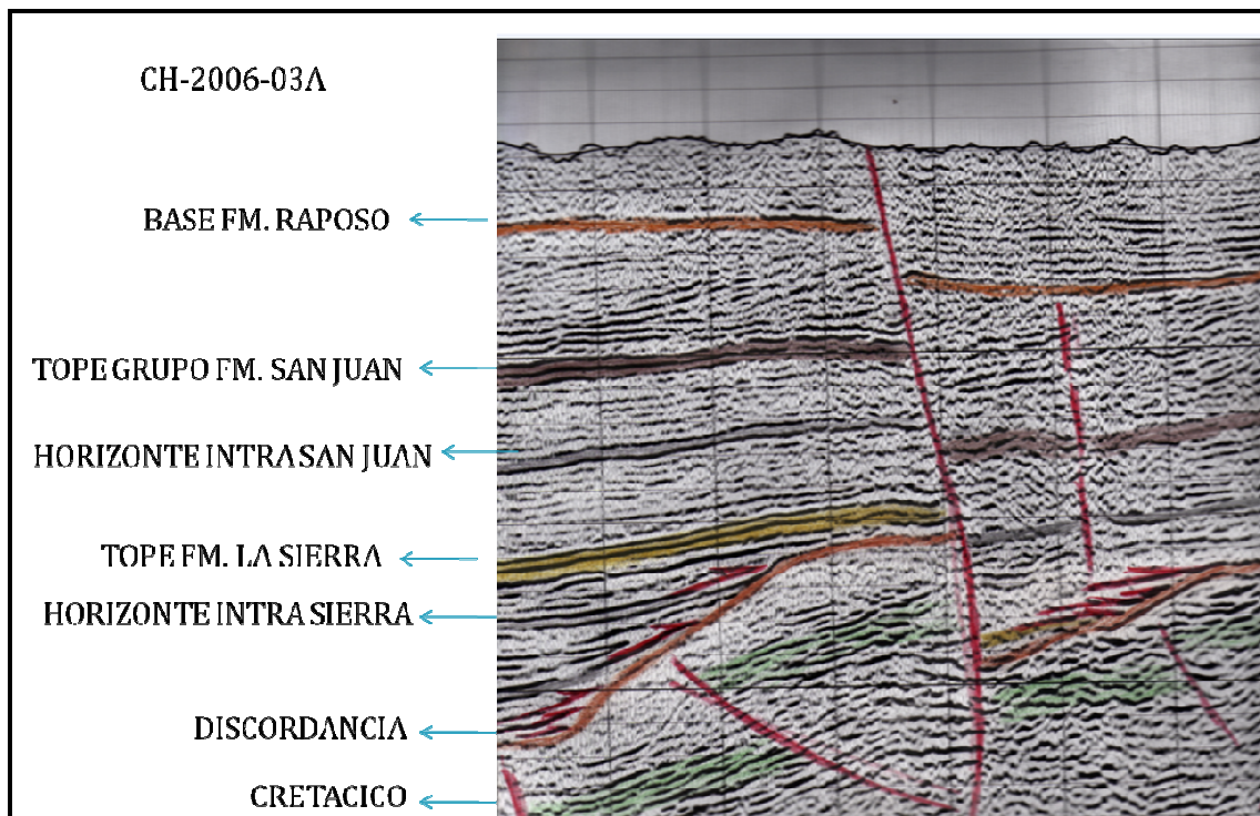
Figura 11. Sección ANH-CH (B) 2006-03A. Horizontes mapeados
