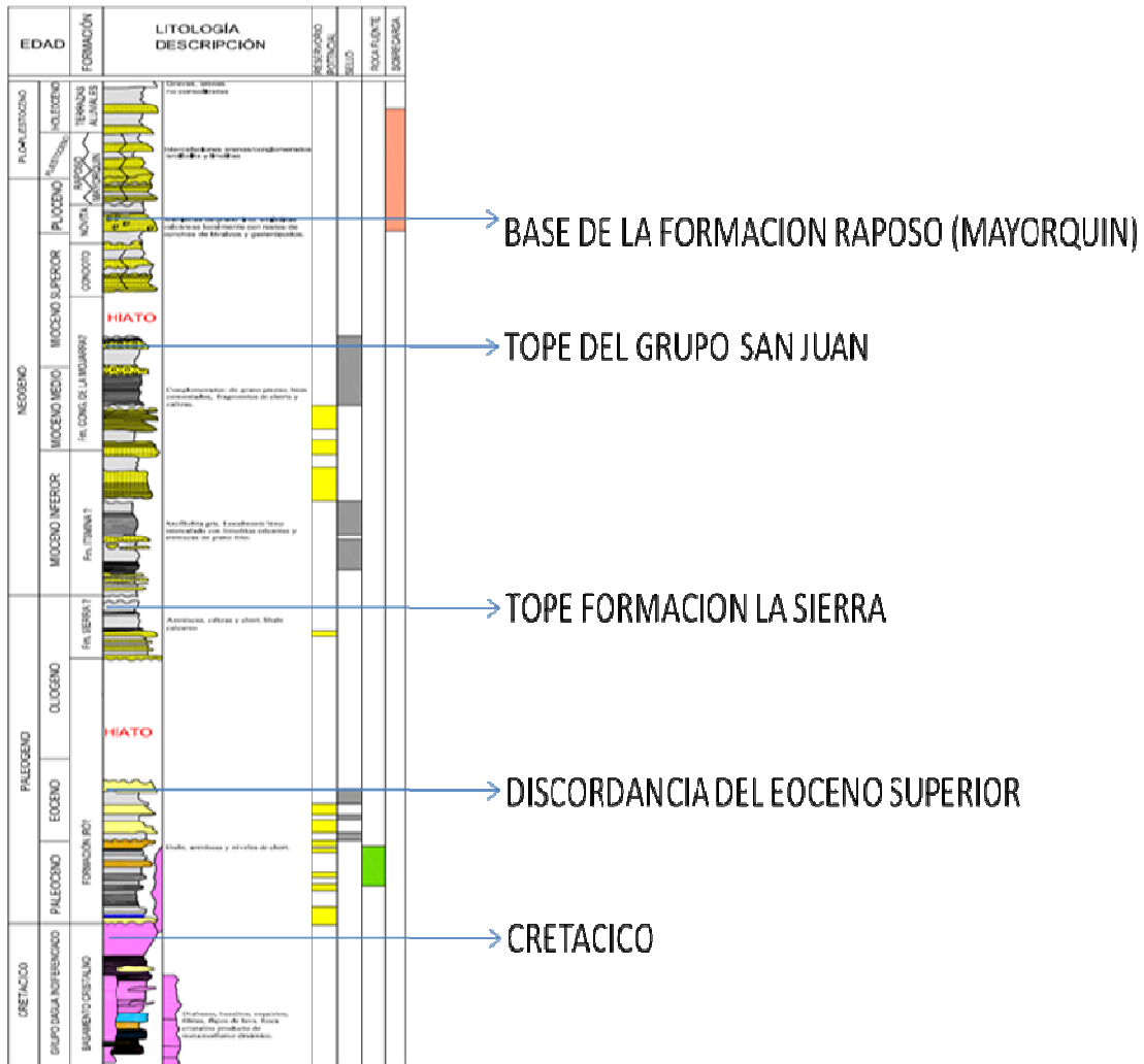
Figura 12. Serie sedimentaria y horizontes mapeados
