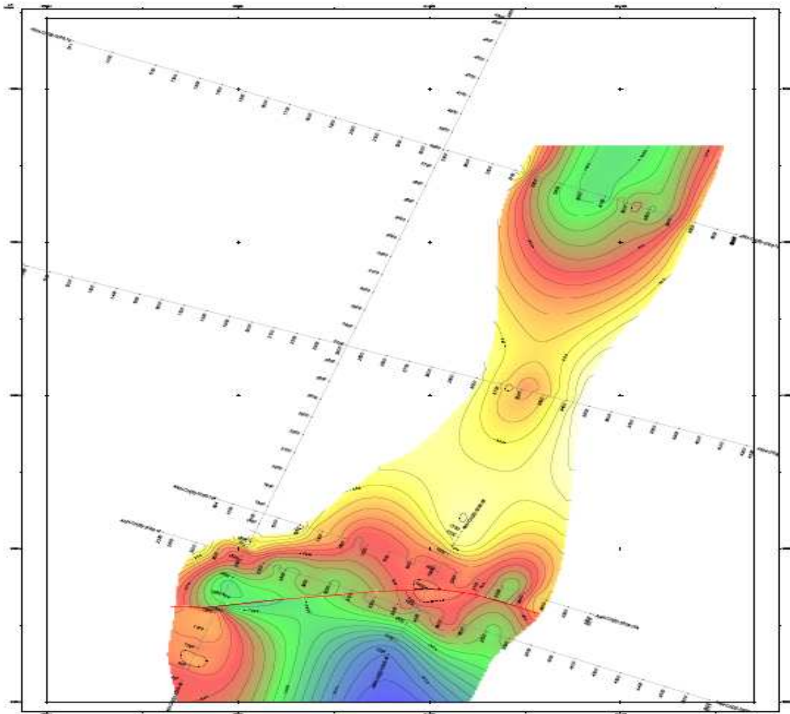
Figura 30. Mapa estructural Base de la Formación Raposo IC: 100 pies
