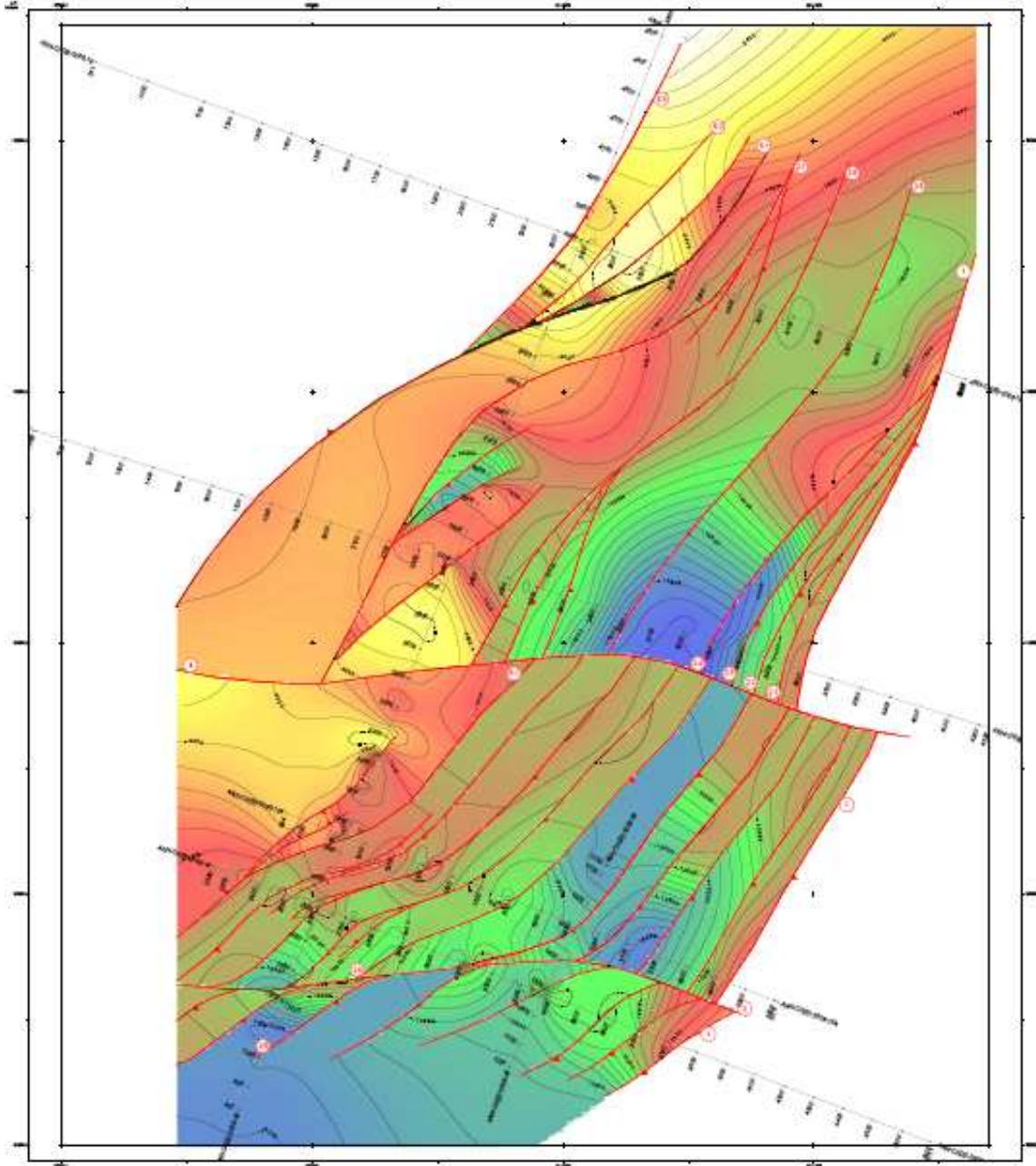
Figura 25. Mapa estructural de basamento IC: 500 pies
