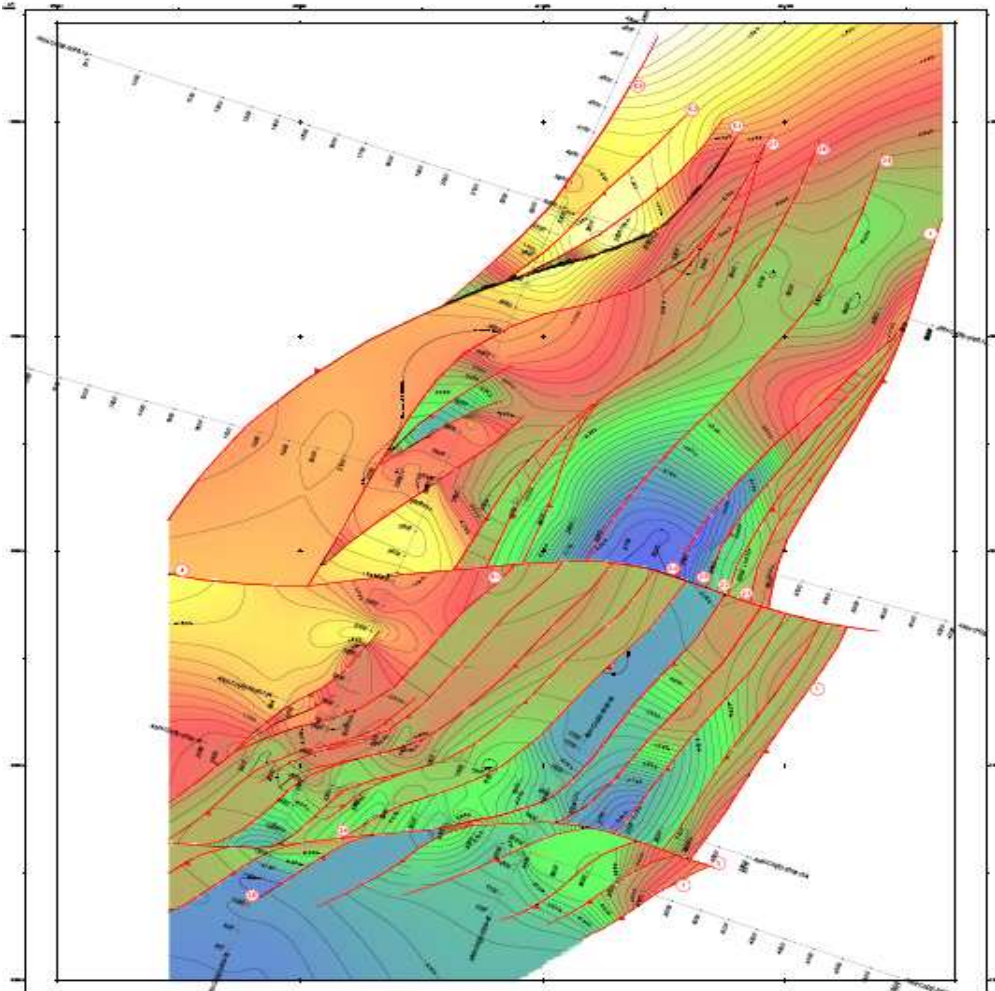
Figura 19. Mapa estructural de basamento TWT. IC: 50 Mlsg. Datum: 500 METROS SNM
