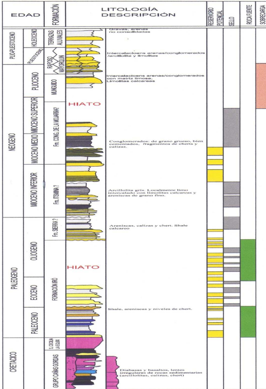
Figura 7. Columna estratigráfica subcuena San Juan Área de estudio – tomado de HGA-
