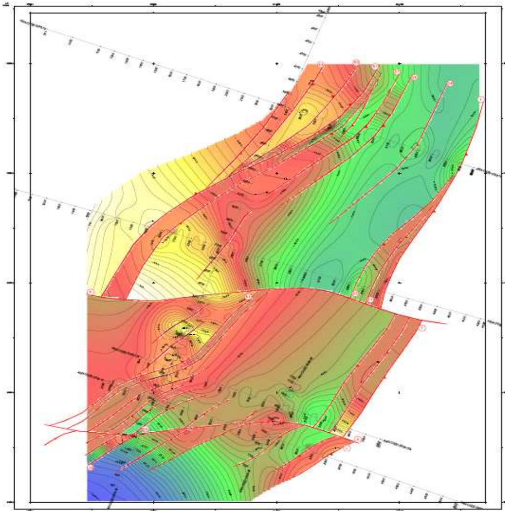
Figura 27. Mapa estructural del Eoceno Medio IC: 200 pies
