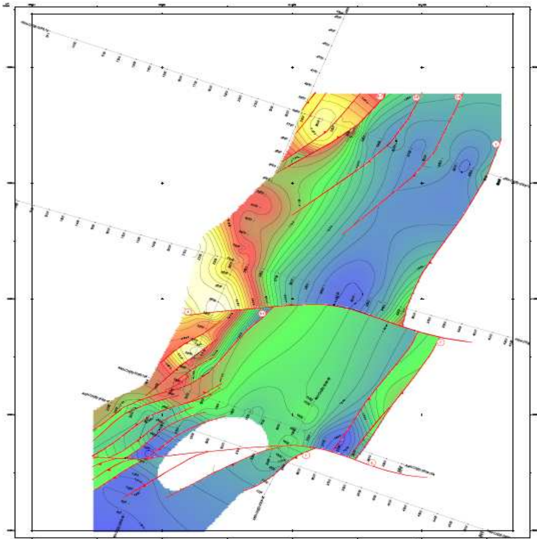
Figura 22. Mapa estructural de la formación La Sierra TWT IC: 100 Mlsg. Datum: 500 metros SNM
