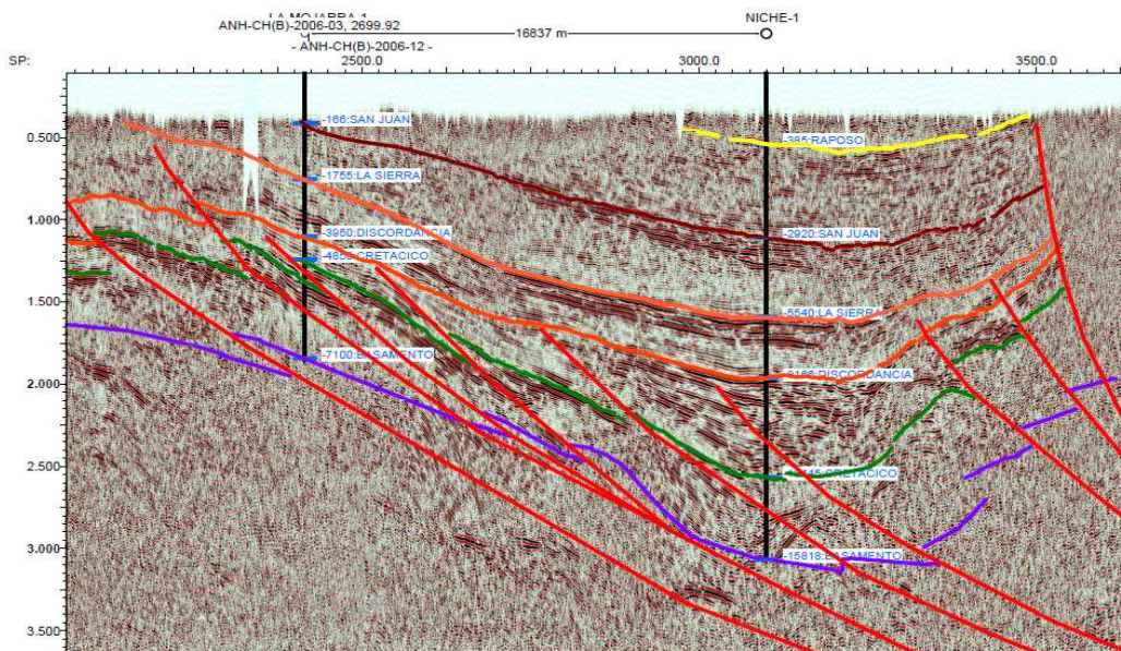
Figura 32. Perfil sísmico con áreas de interés.
