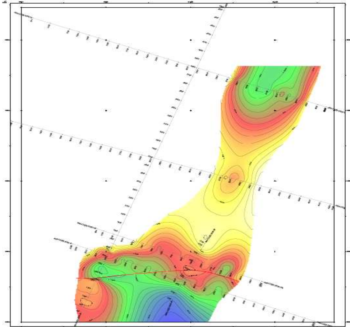
Figura 24. Mapa estructural Base Raposo-Mayorquín TWT IC: 10 Mlsg. Datum: 500 metros SNM
