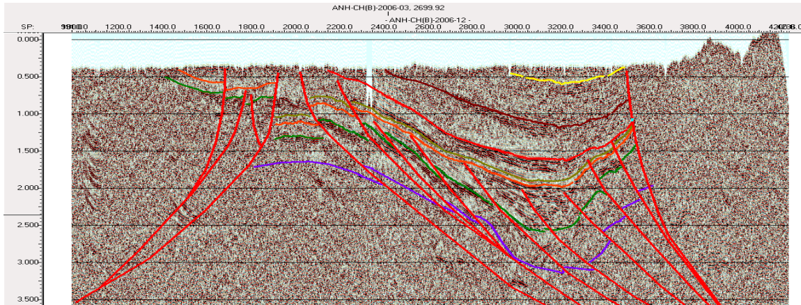
Figura 9. Sección sísmica ANH-CHOCO (B)-2006-12
