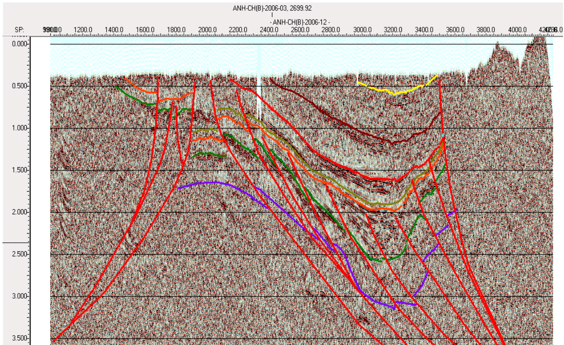
Figura 14. Sección sísmica ANH-CHOCO-2006-12 Migrada en tiempo
