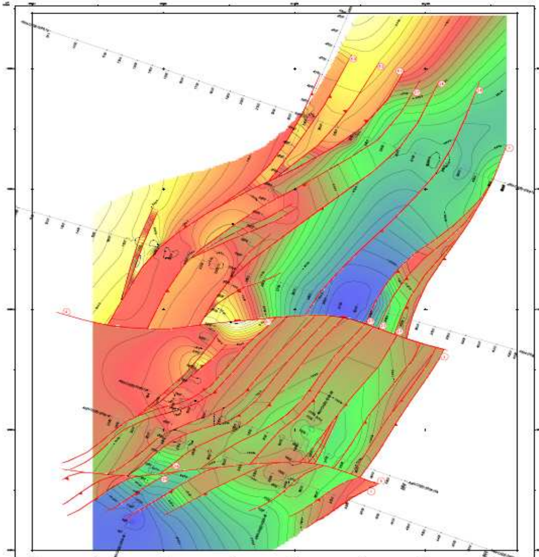
Figura 26. Mapa estructural Cretáceo-Paleoceno IC: 500 pies
