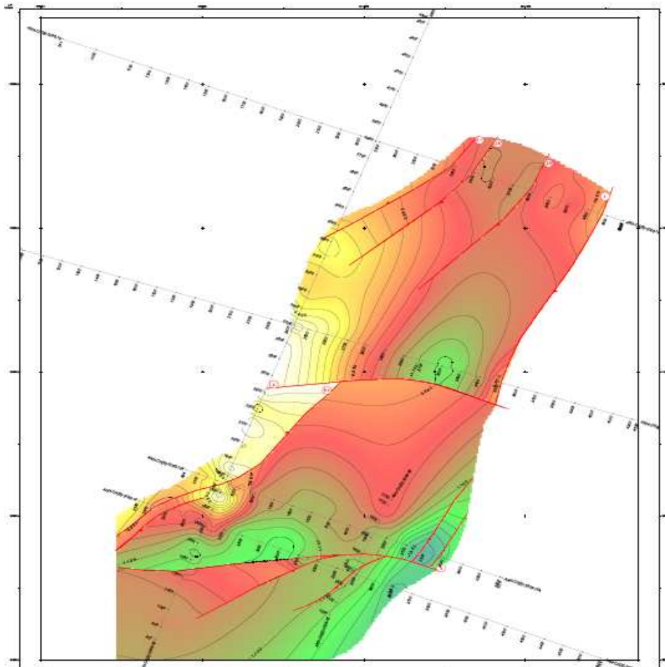
Figura 23. Mapa estructural Tope del Grupo San Juan TWT IC: 100 Mlsg. Datum: 500 metros SNM.
