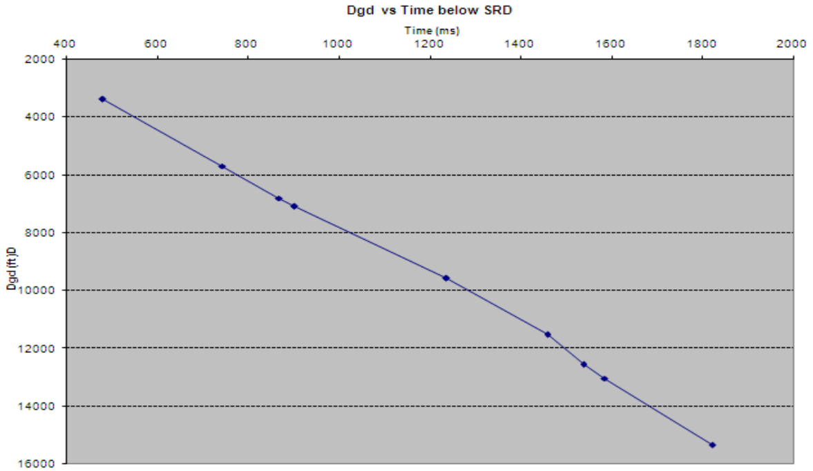
Curva de velocidades obtenida de tiempo Vs Profundidad en Buchado-1
