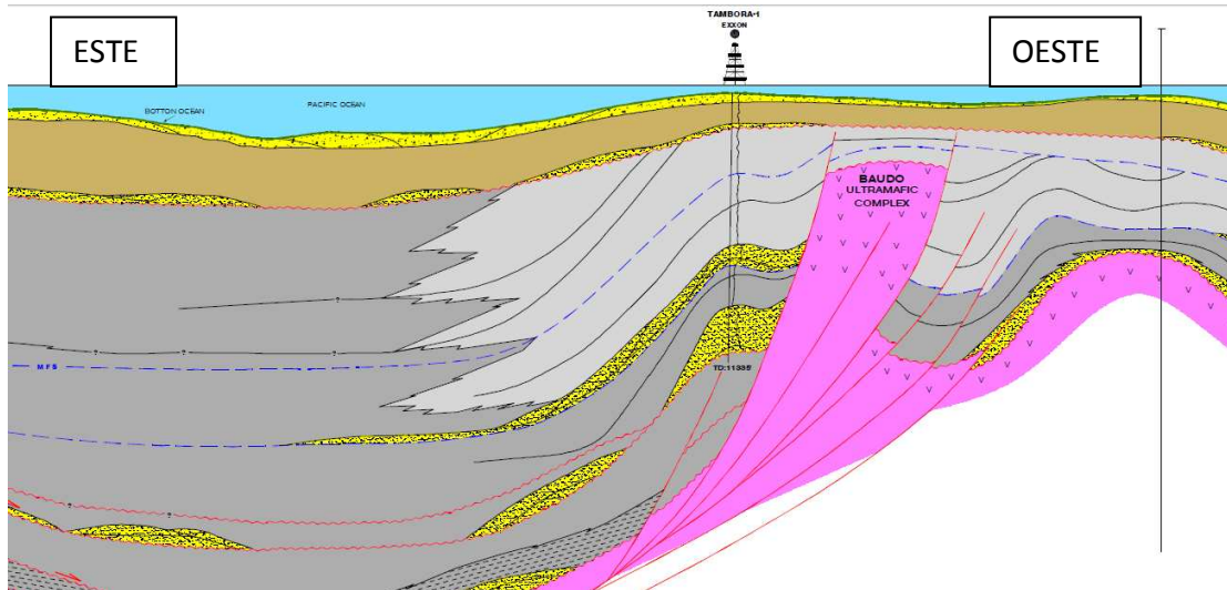
Figura 3A. Modelo de estructura en la perforación de Tambora-1
