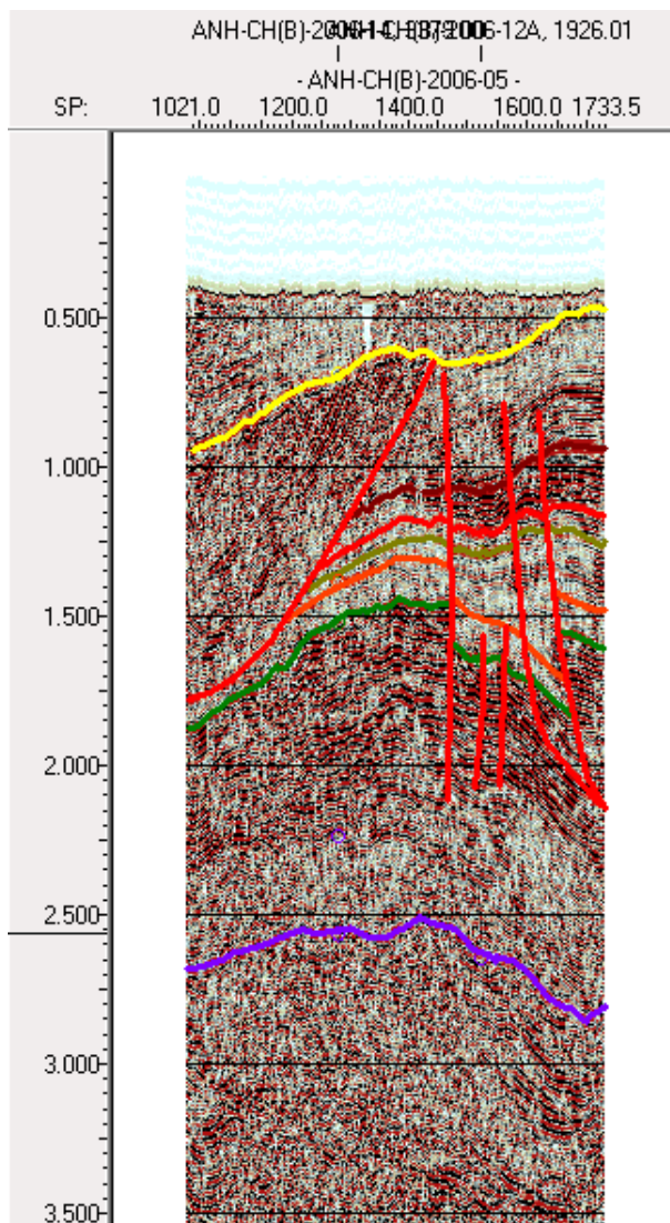
Figura 18. Sección sísmica ANH-CHOCO (B)-2006-05 Migrada en tiempo.
