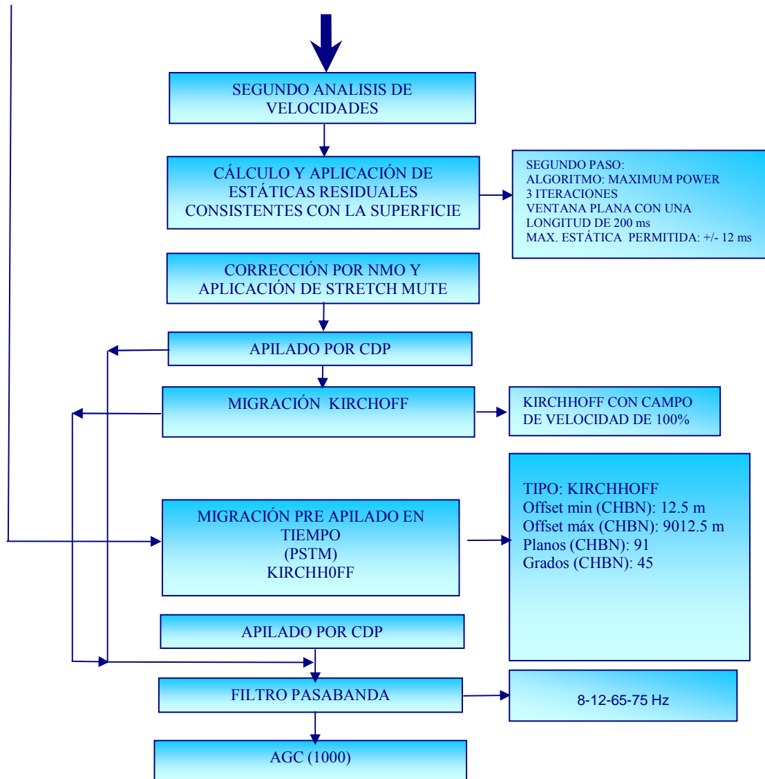
Figura 3. Secuencia de Proceso del Programa Sísmico ANHCHBN 2D-2005
