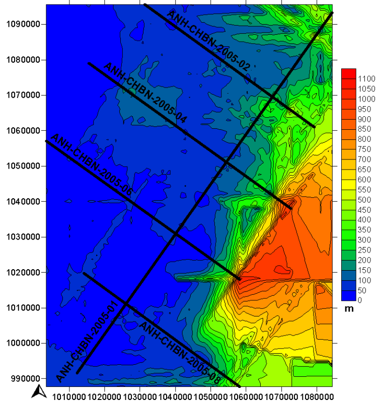
Figura 5. Mapa de Elevaciones Campaña ANHCHBN 2D-2005.
