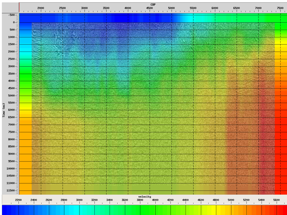
Figura 8. Campo de Velocidades Correspondiente a la línea ANHCHBN-2005-04Programa ANHCHBN 2D-2005.
