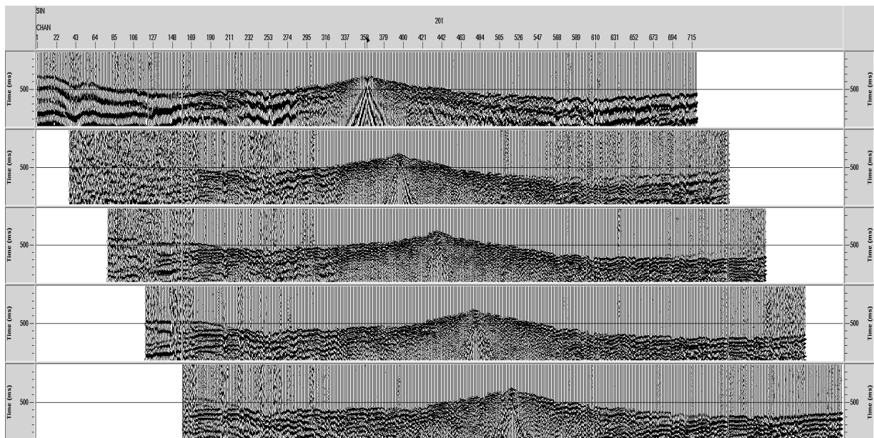
Figura 4. Revisión de Geometría por Corrección de Lineal Moveout.
