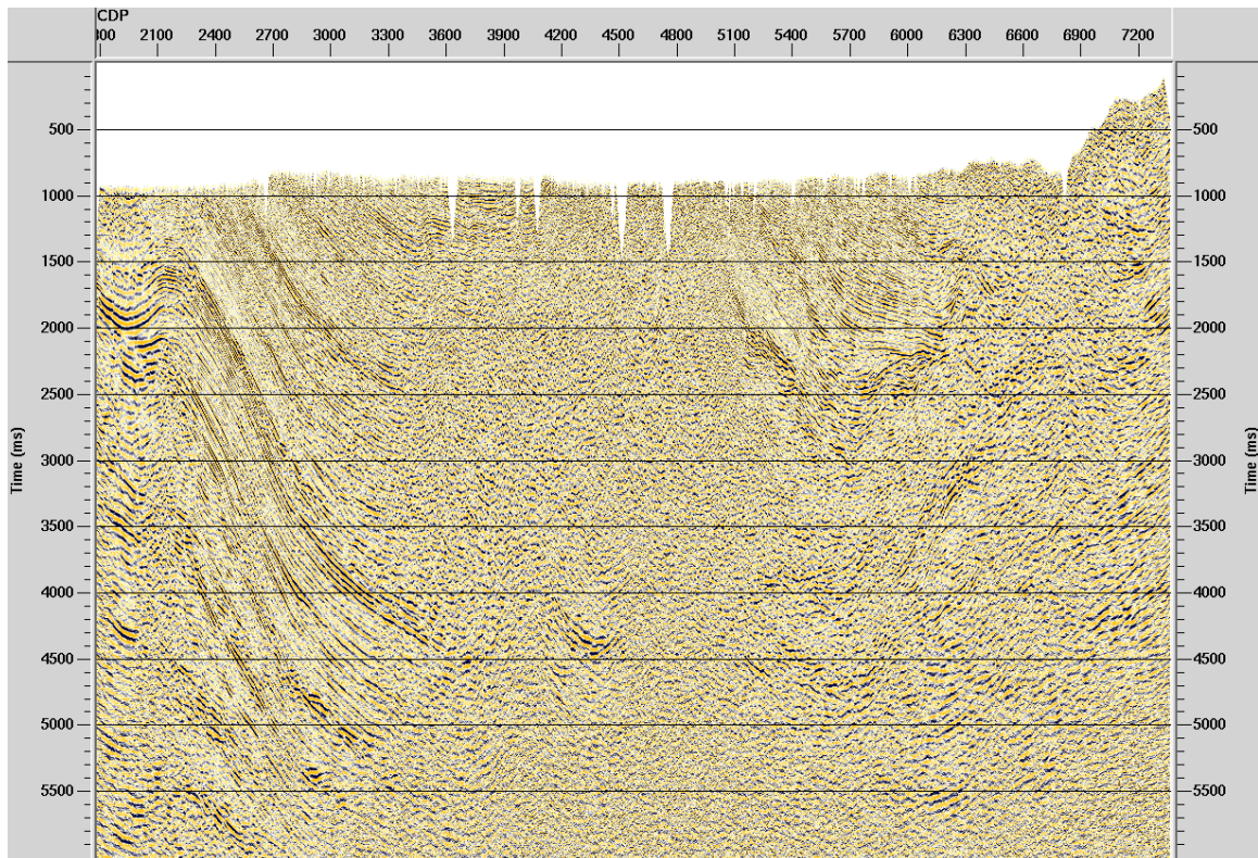
Figura 16. Migración Pre-Apilado en tiempo línea ANHCHBN-2005-04 con FX-Decon.
