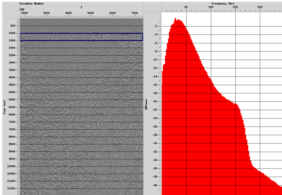
Figura 12. Espectro de frecuencia apilado parte somera.
