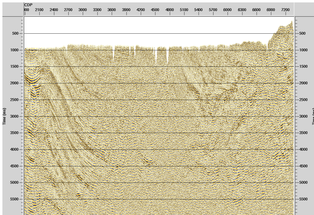
Figura 15. Migración Pre-Apilado en tiempo línea ANHCHBN-2005-04 sin FX-Decon.
