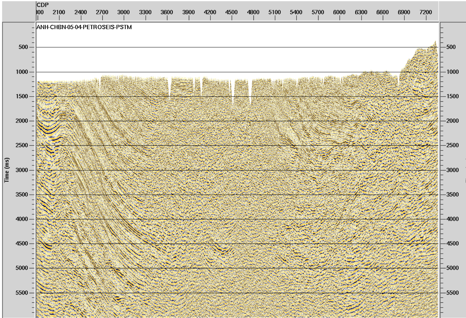
Figura 9. Migración PSTM Correspondiente a la línea ANHCHBN-2005-04 Programa ANHCHBN 2D-2005.
