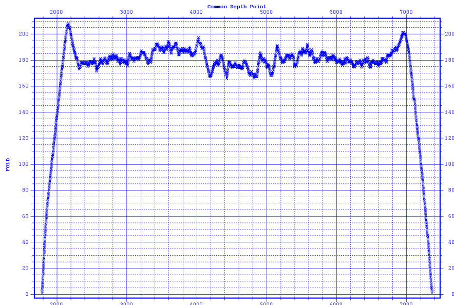
Figura 6. Diagrama de Cubrimiento Campaña ANHCHBN 2D-2005
