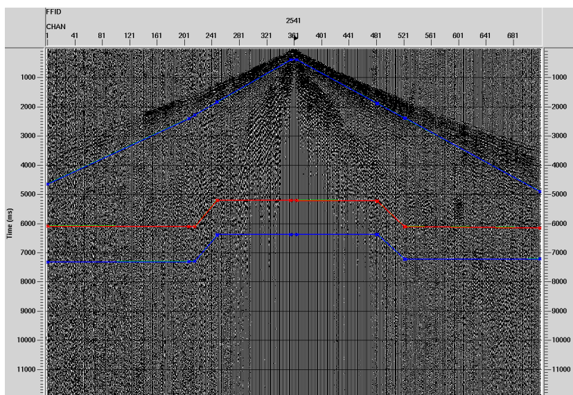
Figura 7. Ventanas de deconvolución Campaña ANHCHBN 2D-2005.
