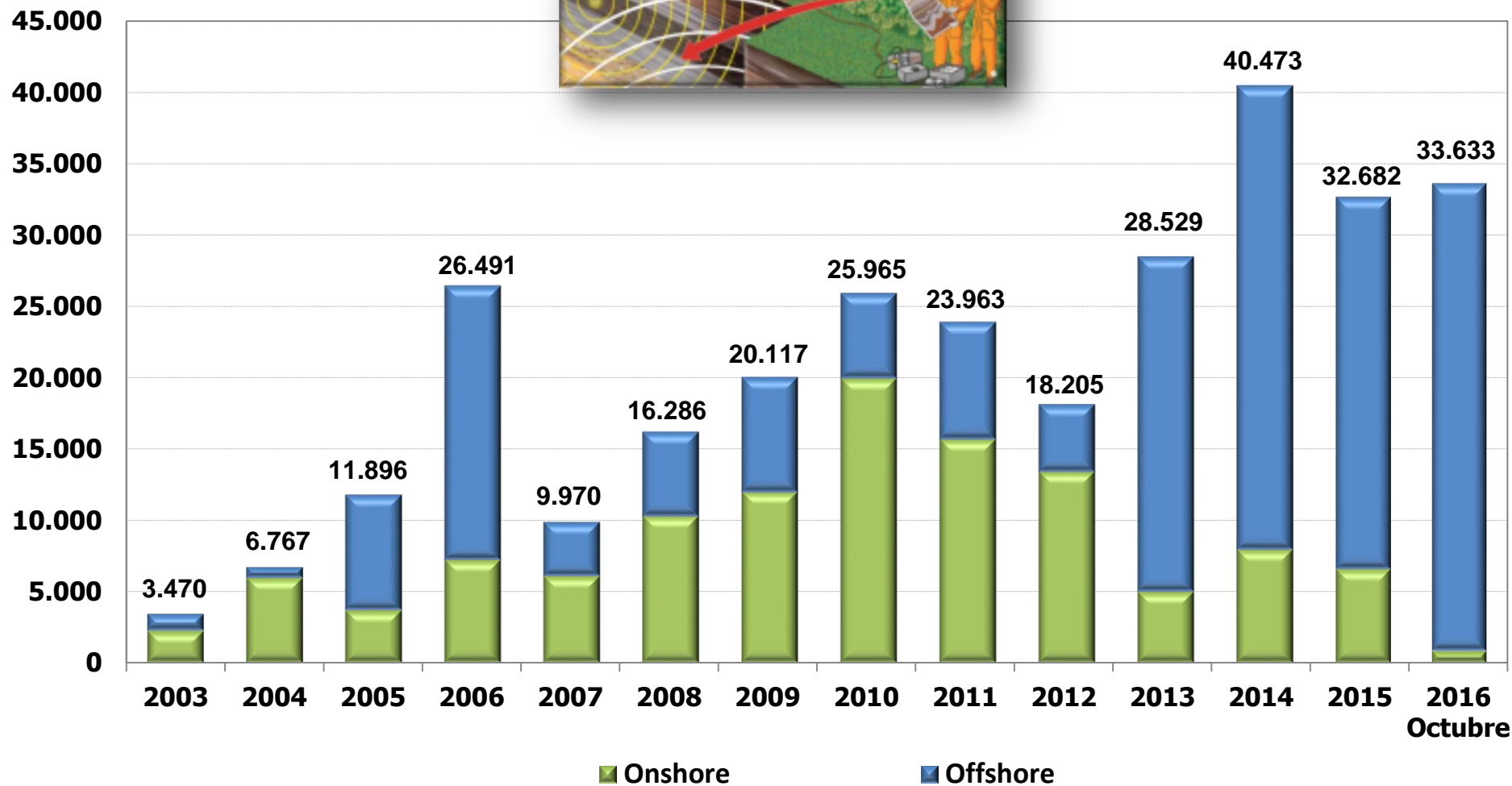
km de sísmica 2D equivalente
