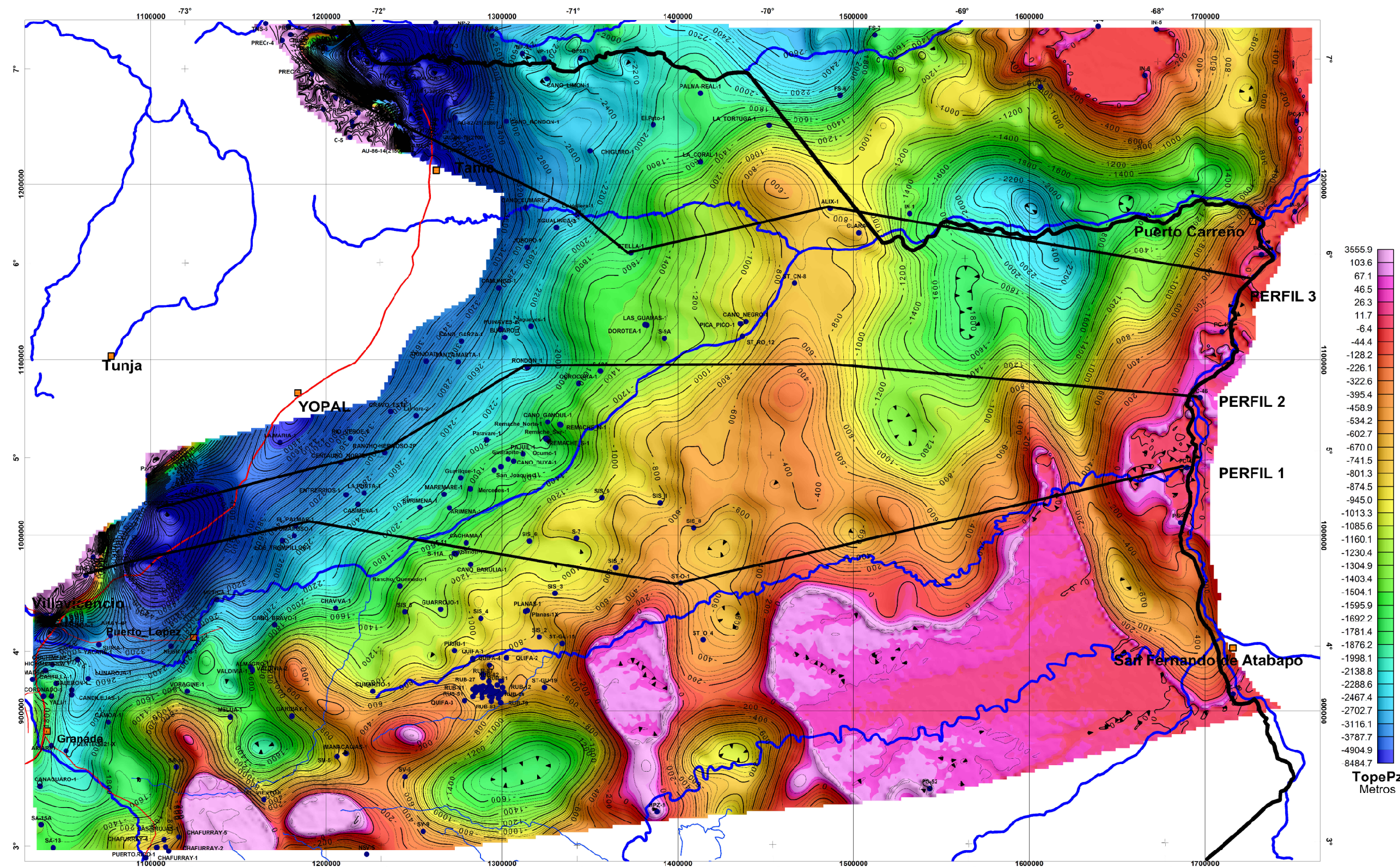
Topo del Paleozoico (Inversión 3D del Residuo Controlado)
