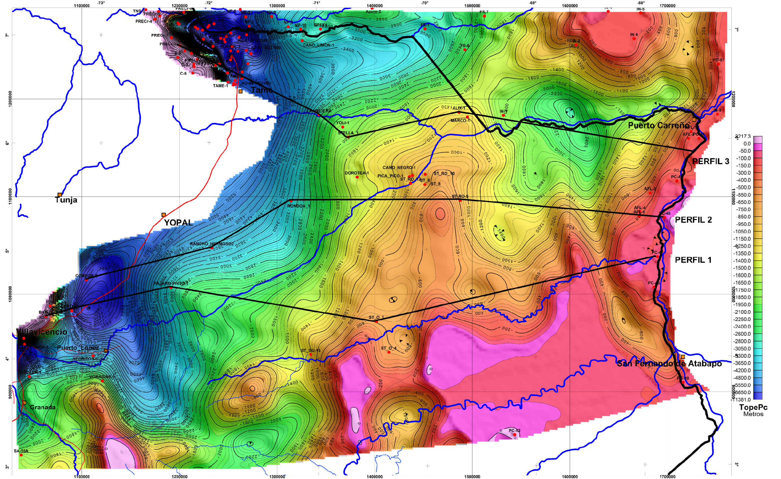
Topo del Basamento Precámbrico (Inv. 3D del Residuo Controlado)
