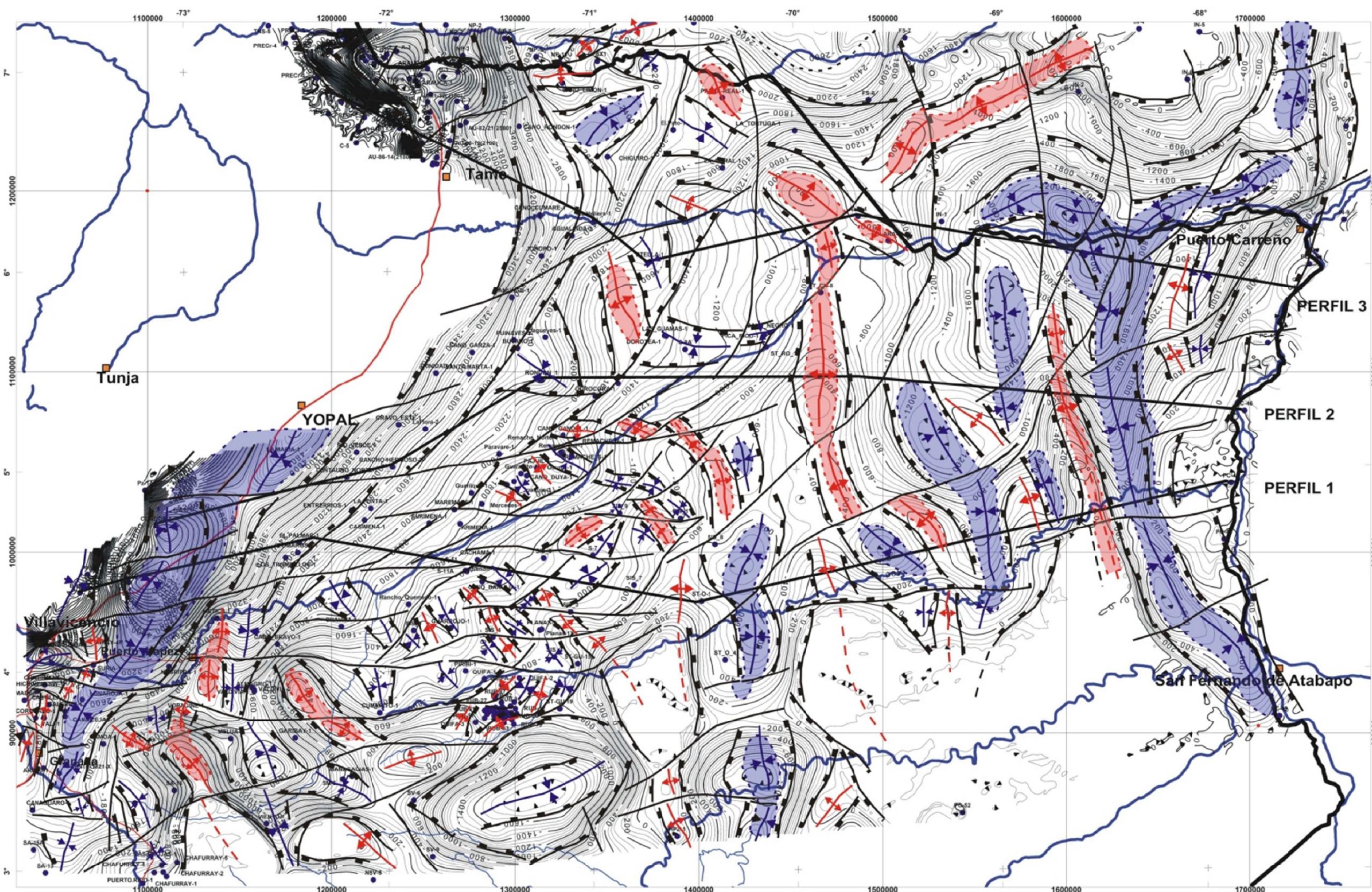
Interpretación Estructural Topo del Paleozoico
